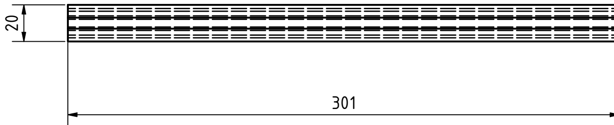
VIEW2 ( 2 : 1 )
